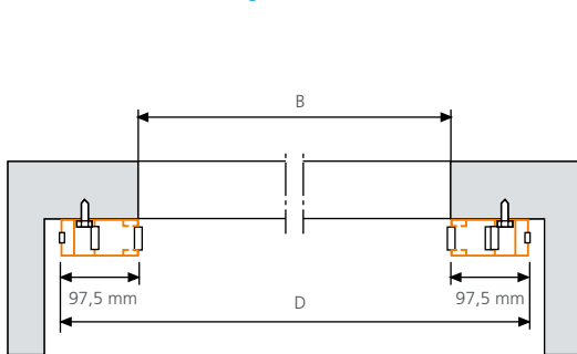
Einbau hinter dem Anschlag montiert
