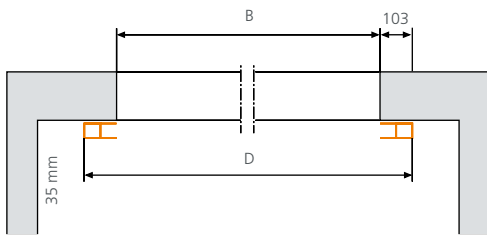
Einbau Rechtsroller – innen hinter der Laibung montiert
