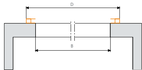
Einbau Linksroller – aussen auf das Mauerwerk montiert
