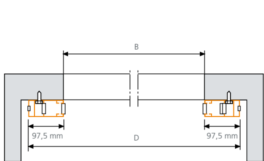
Installation montée derrière la butée
