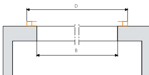
Installation roulette à gauche – montée à l'extérieur sur la maçonnerie
