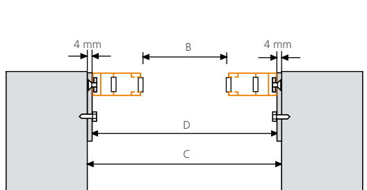
Installation montée sans butée
