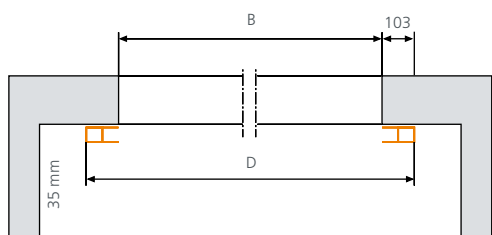
Installation roulette à droite – montée à l'intérieur derrière l'embrasure
